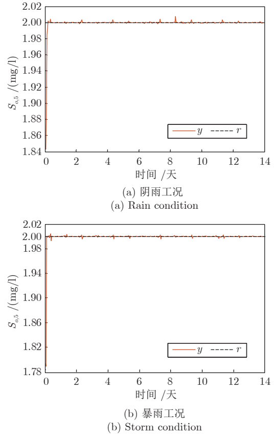
图5 恒定 S_o 控制效果
