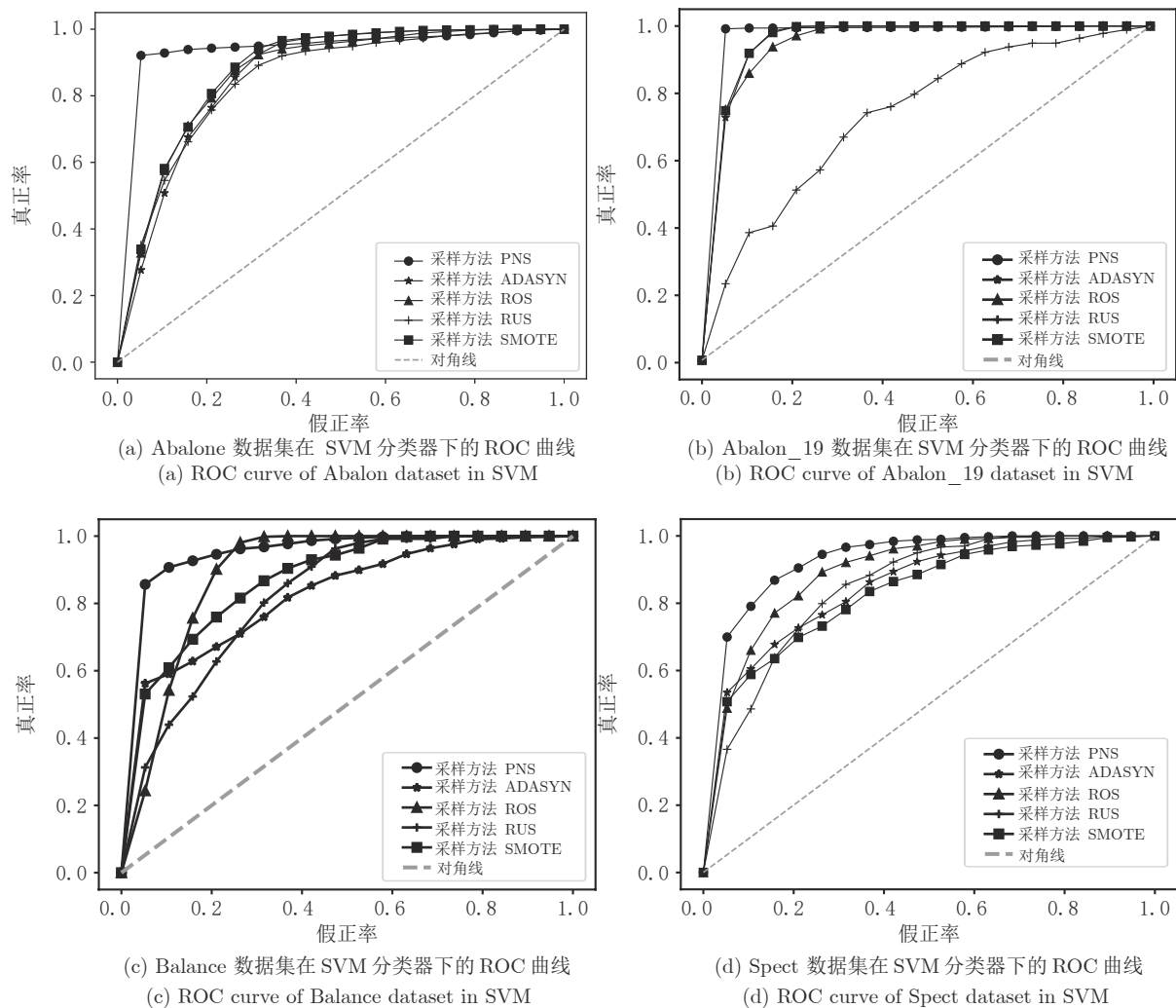
图 2 4 个 UCI 数据集在 SVM 分类器下的 ROC 曲线
