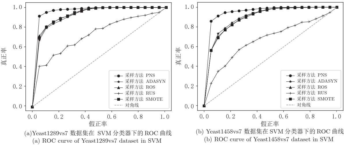
图 3 2 个 KEEL 数据集在 SVM 分类器下的 ROC 曲线 Fig.3 ROC curve of two KEEL datasets in SVM classifier
