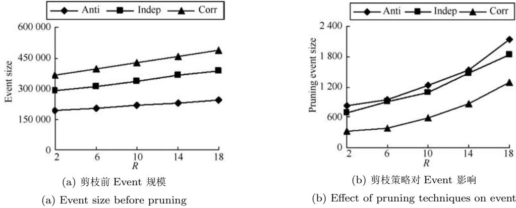
图 9 R 在圆形-均匀分布模型中对 Event 的影响
