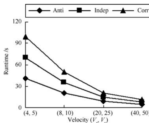
(b) U_SPSC 算法的运算时间
