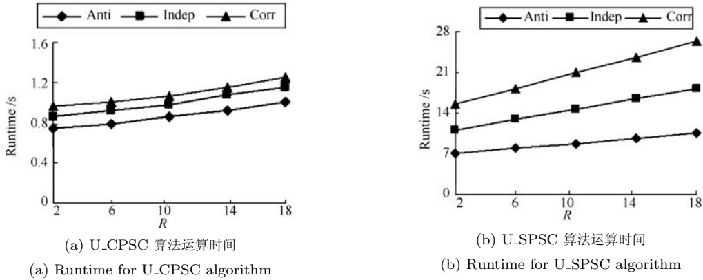
图 10 R 在圆形-均匀分布模型中对算法运行时间的影响
