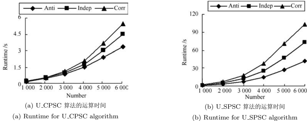
图 5 数据规模在圆-均匀分布 (Circle-uniform) 模型中对算法运行时间的影响
