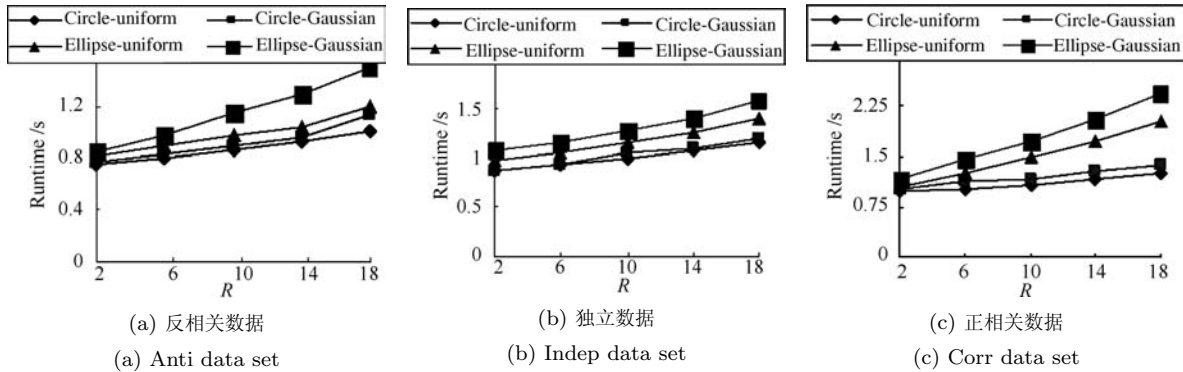
图 11 R 在不同模型中对算法运行时间的影响
