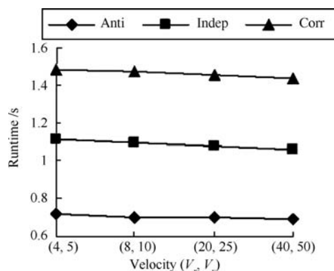
(a) U_CPSC 算法的运算时间
