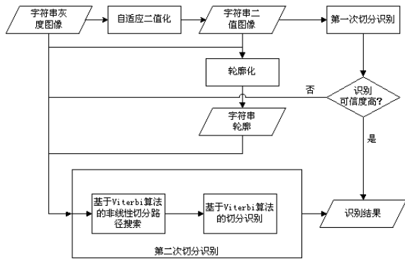
图 1 切分识别系统流程图
