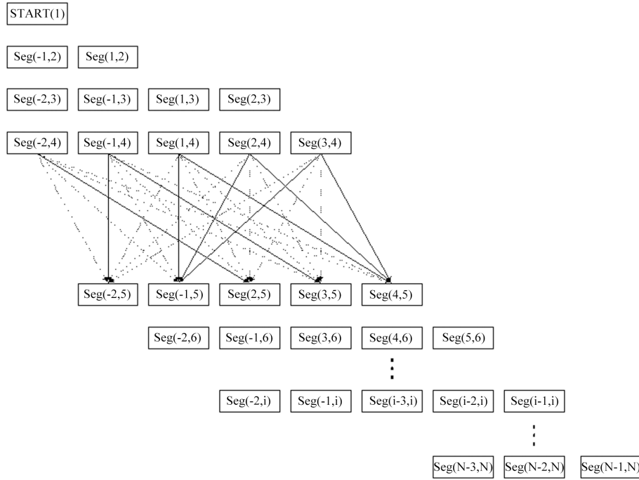
图 4 N 个候选切分点的切分情况图
