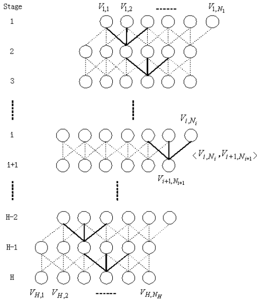
图 2 切分区的图表示 [3]
