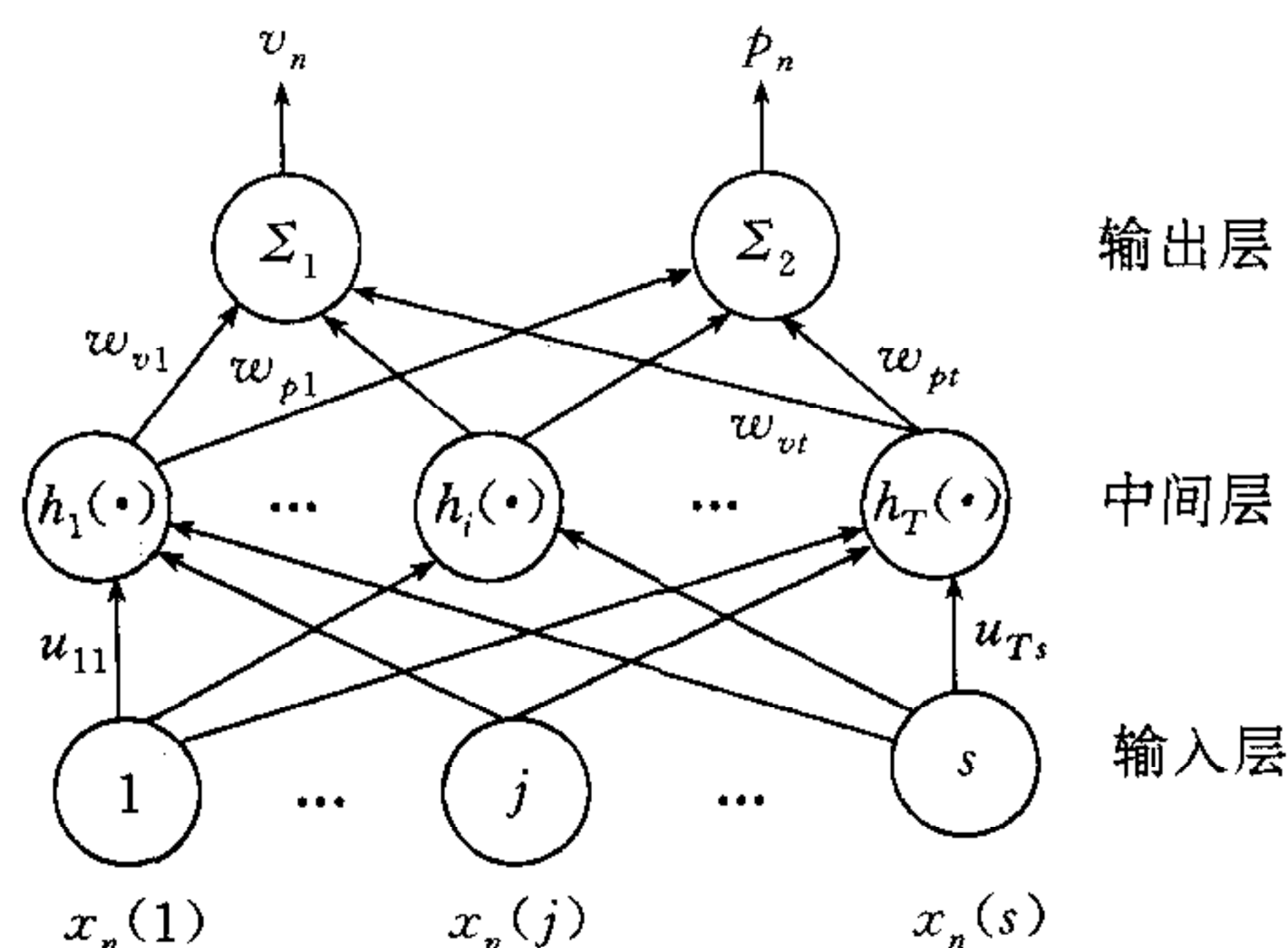
图 1 小波神经网络结构
