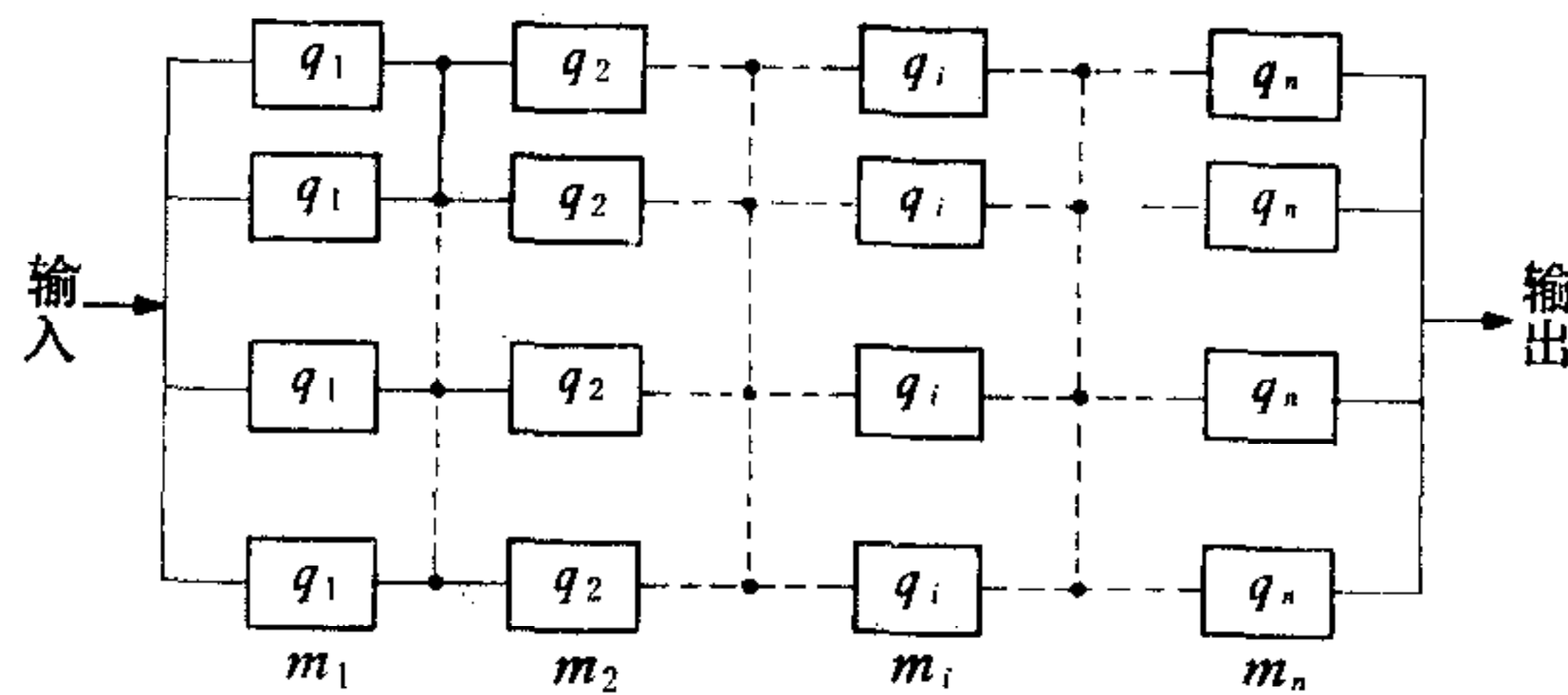
图 1 可靠性串并联复式系统
