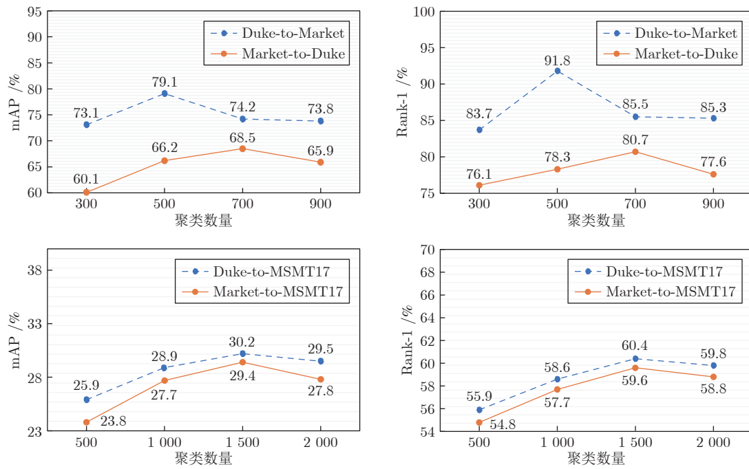
图 5 聚类数量取值评估实验
