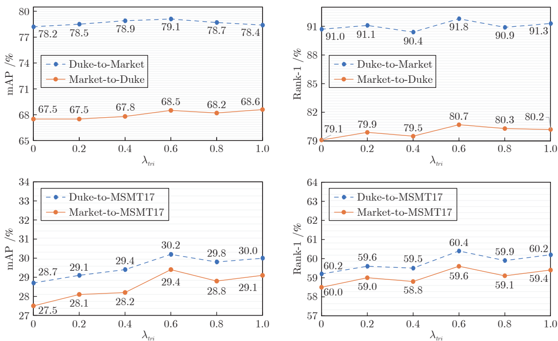
图 4 \lambda_{tri} 取值评估实验
