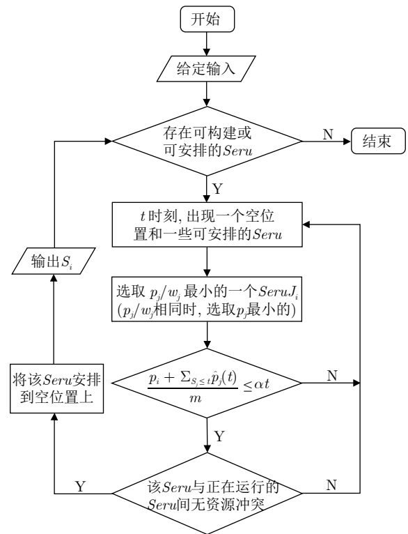
图 5 \alpha AD-I 算法流程图
