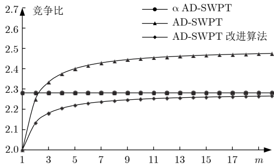
图 4 三个算法的竞争比
