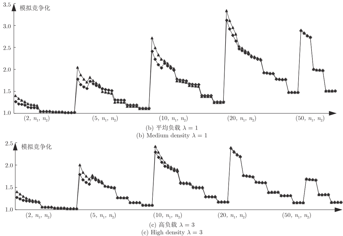
图9 \alpha AD-I算法与AD-SWPT改进算法在一般实例下的实验结果对比
