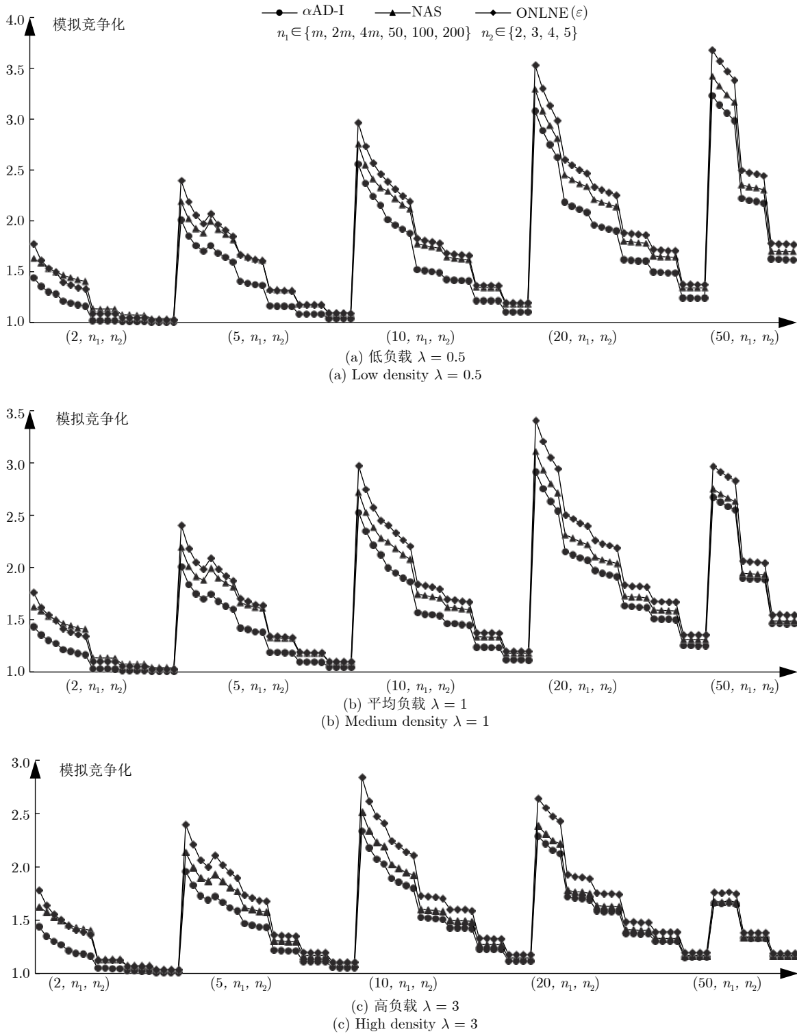
图 6 \alpha AD-I 算法在特殊实例 I^* 下的实验结果 Fig.6 The experimental results of \alpha AD-I in I^*
