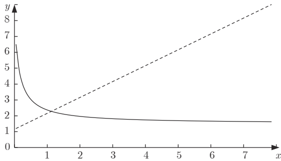
图 3 f(\alpha) 与 g(\alpha) 的图像 Fig.3 Graphs of f(\alpha) and g(\alpha)
