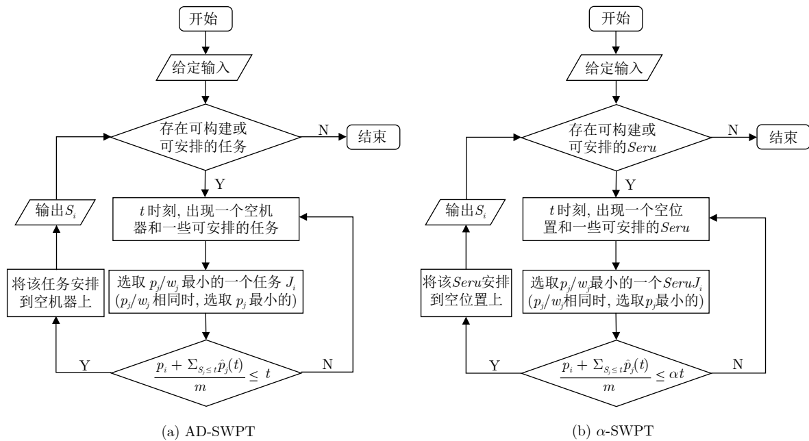
图 1 AD-SWPT 与 \alpha AD-SWPT 算法流程图 Fig. 1 The flow charts of AD-SWPT and \alpha AD-SWPT
