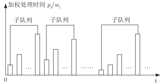
图 2 按照 \alpha AD-SWPT 安排方案的构建时间示意图 Fig.2 Processing sub-queues in terms of starting time in the \alpha AD-SWPT schedule
