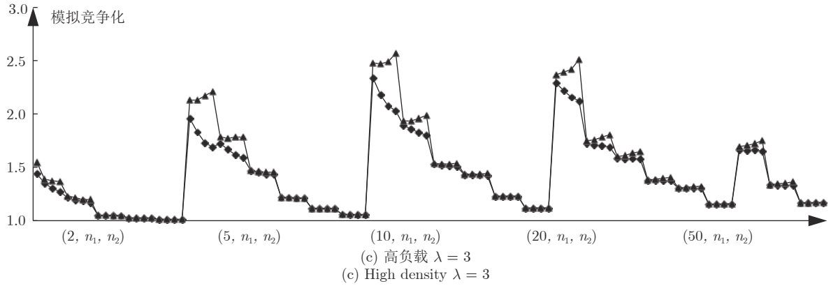
图 8 \alpha AD-I 算法在 T 与一般实例下实验结果对比
