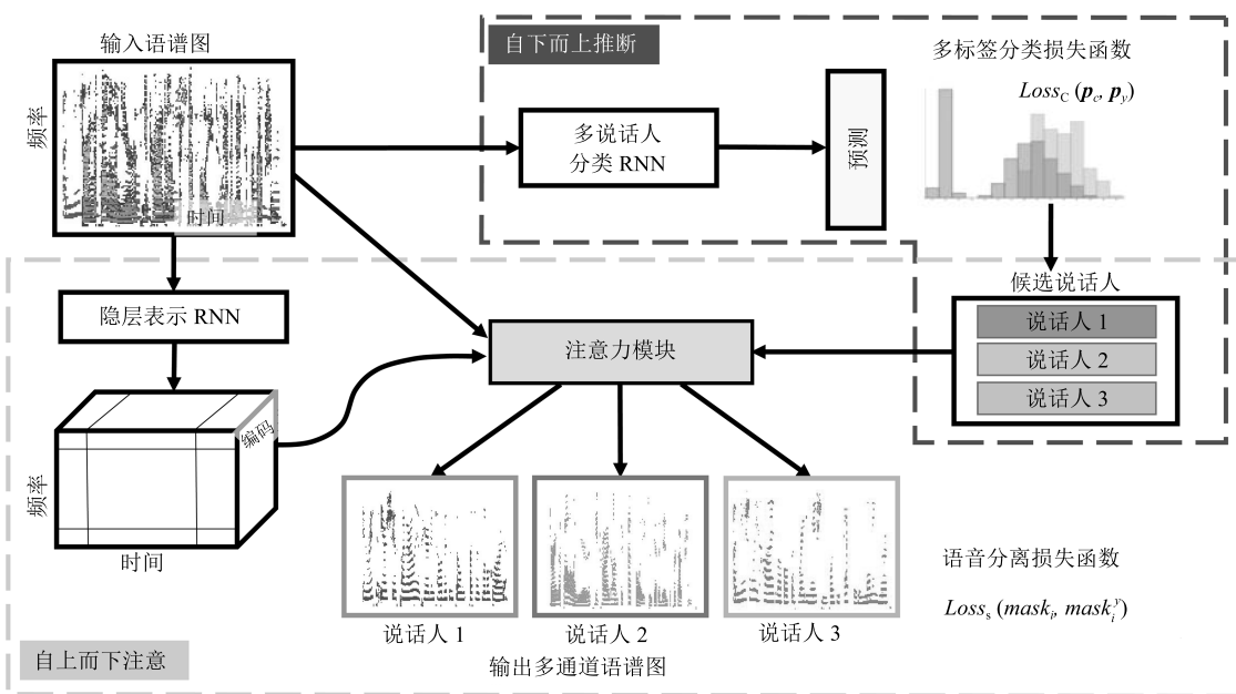
图 5 Shi 等提出的 TDAA 系统的结构 [96]
