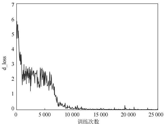
图 10 MNIST 上 d_loss 变化趋势 (PrimaryCaps 层胶囊个数为 24)
