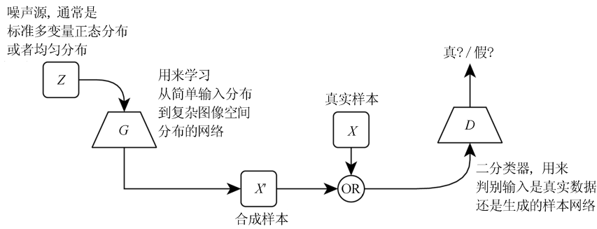
图 1 GAN 架构图
