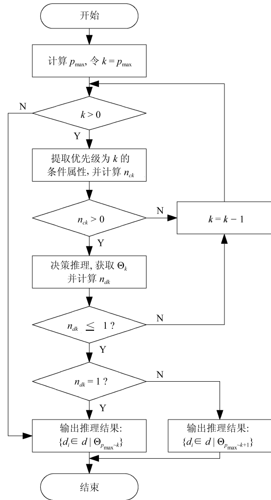
图 4 RBFLR 方法流程图
