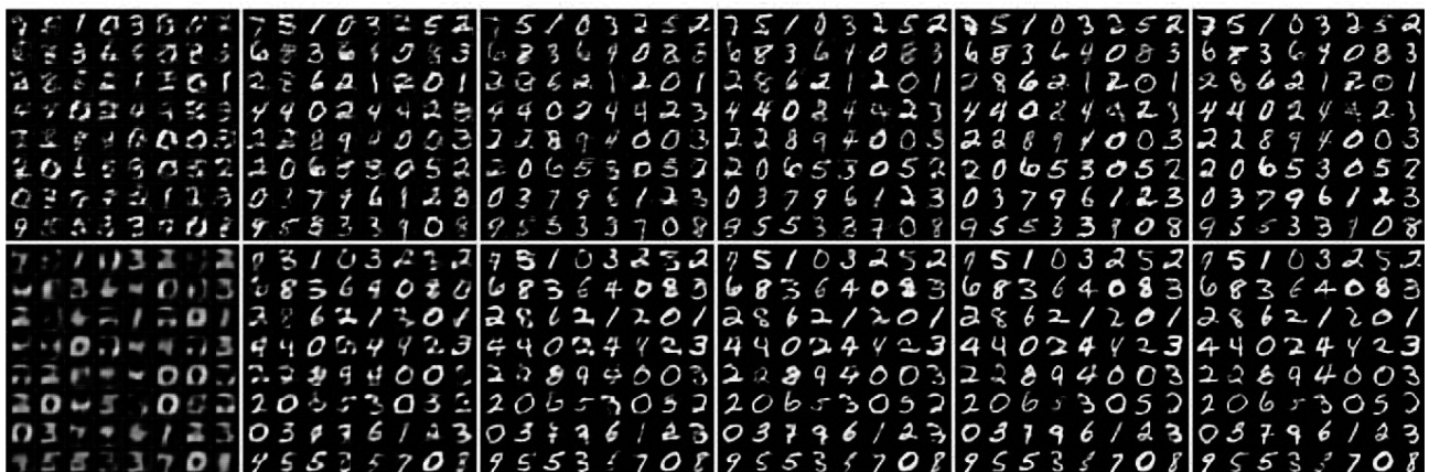
(a) 迭代 200 次 (b) 迭代 500 次 (c) 迭代 1000 次 (d) 迭代 2000 次 (e) 迭代 4000 次 (f) 迭代 6000 次 (a) 200 iterations (b) 500 iterations (c) 1000 iterations (d) 2000 iterations (e) 4000 iterations (f) 6000 iterations
