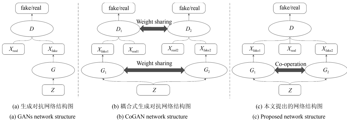
图 2 网络结构图 Fig. 2 Network structure
