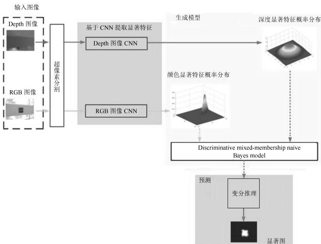
(b) 预测阶段, 基于 DMNB 模型的变分推理进行 3D 显著性预测
