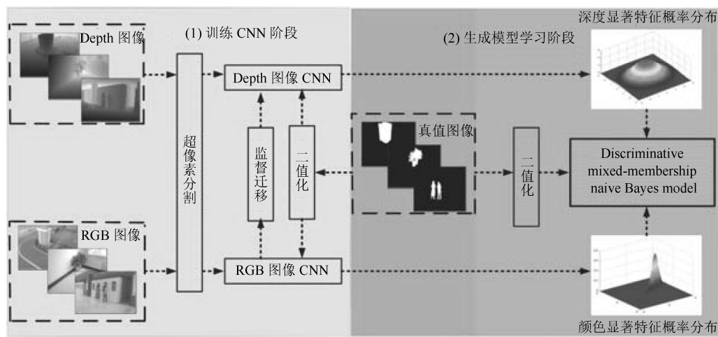
(a) 训练阶段, 包括基于监督迁移的 Depth 图像深层卷积神经网络的训练阶段和 DMNB 生成模型的学习阶段
