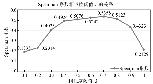
图 8 Spearman 系数与相似度阈值 \lambda 的关系
