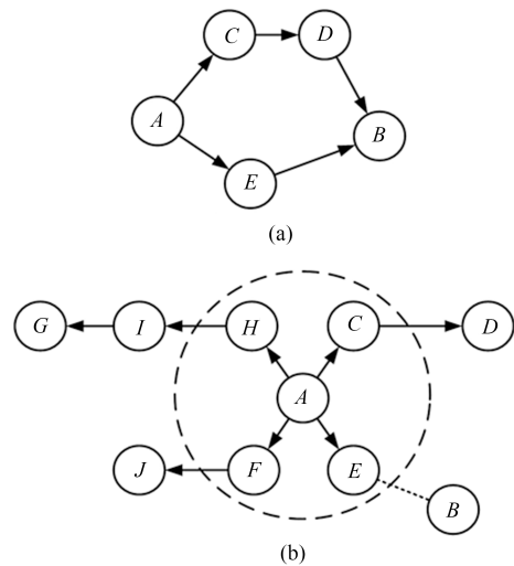
图 2 语义关系图中的语义相关
