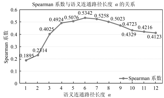
图 7 Spearman 系数与语义连通路程长度 \alpha 关系
