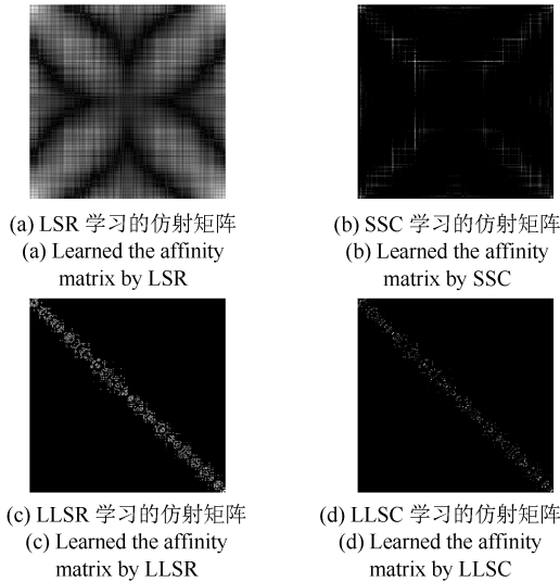
图 4 双月形数据上的仿射矩阵 Fig. 4 The affinity matrixes on the two-moon synthetic data
