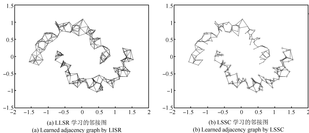
图 3 LSC 在双月形数据学习得到的邻接图
