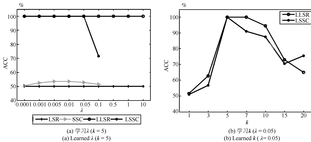
图 5 在双月形数据上 LSC 的参数学习 Fig. 5 Study on the LSC's parameters on the two-moon synthetic data
