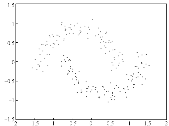
图 2 双月形数据
