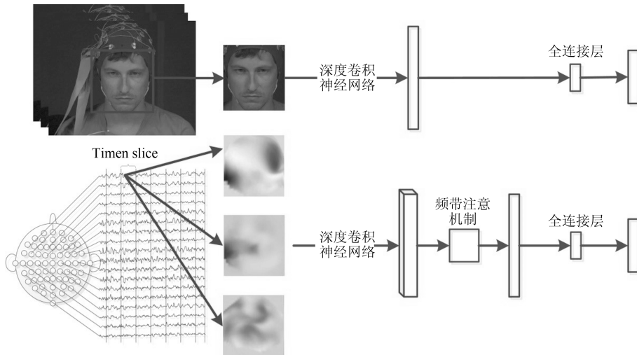
图 3 人脸视频与脑电信号的特征提取过程
