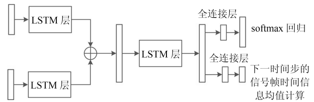
图6 基于 LSTM 与注意机制的交互协同过程
