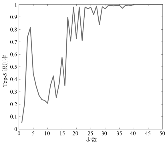
(b) Top-5 识别率
