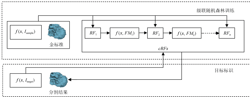
图 3 级联架构下的体素分类流程图
