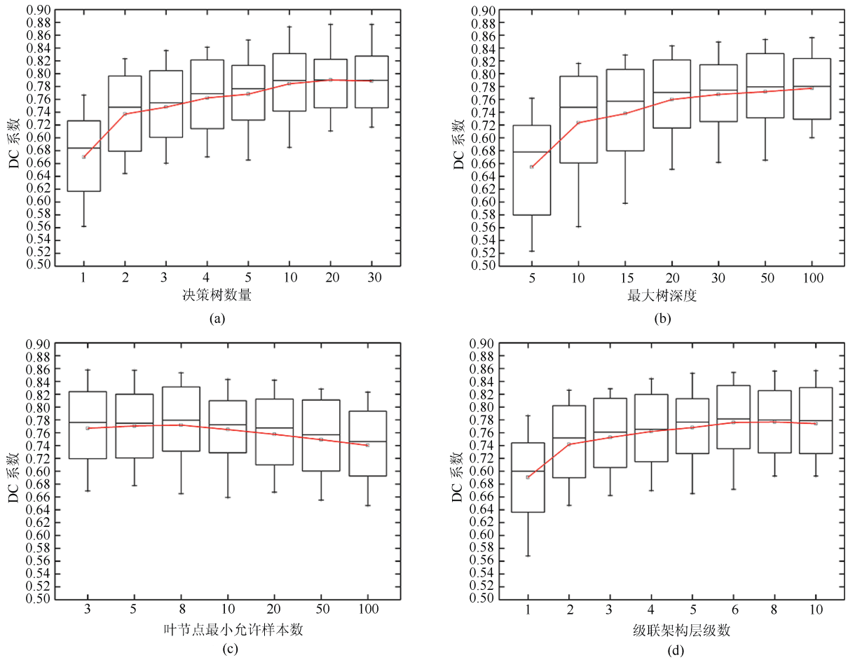
图 7 级联随机森林不同参数对分割结果的影响
