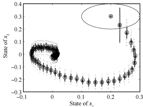
图 5 椭球可行集
