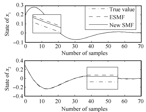
图 3 状态估计
