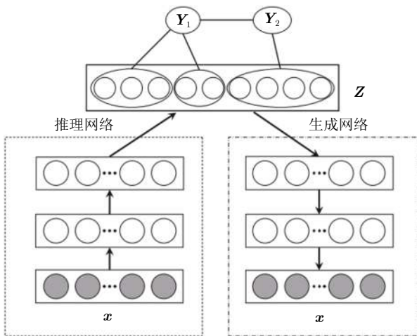
图 7 简易树形变分自编码器模型示意图 [73]
