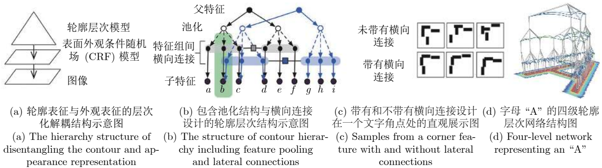
图 8 RCN 模型示意图 [74] Fig. 8 Structure of the RCN [74]
